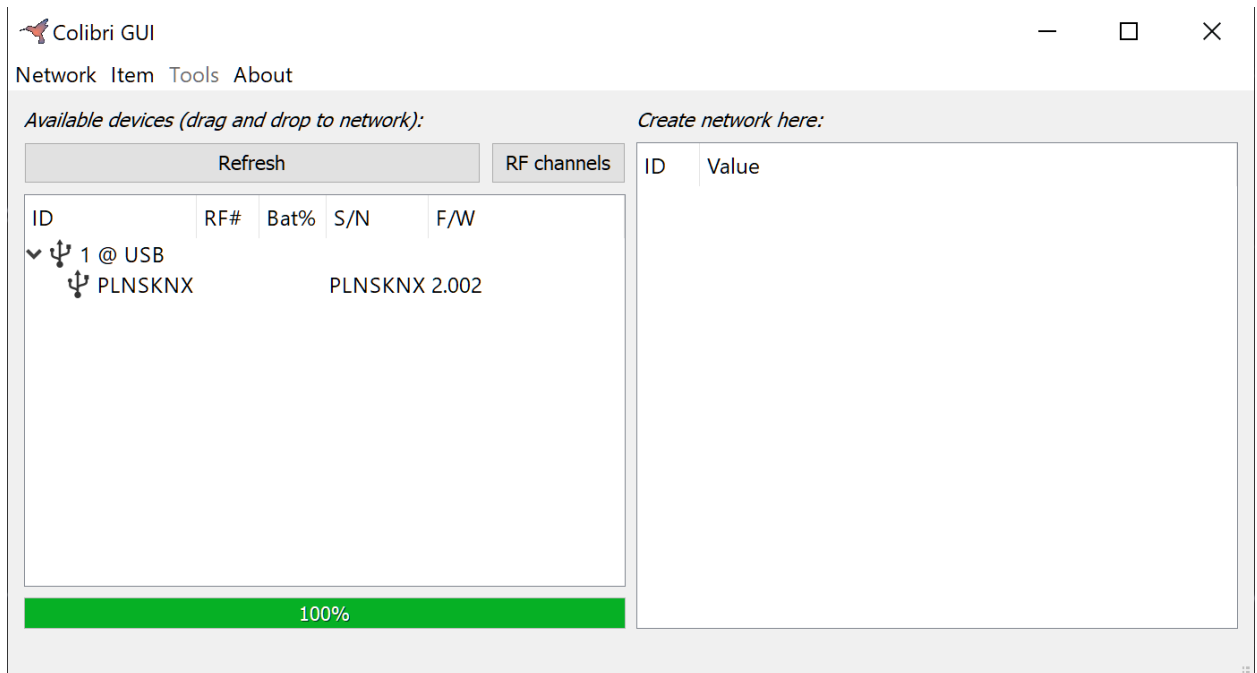
Fig. 1 – Colibri GUI
